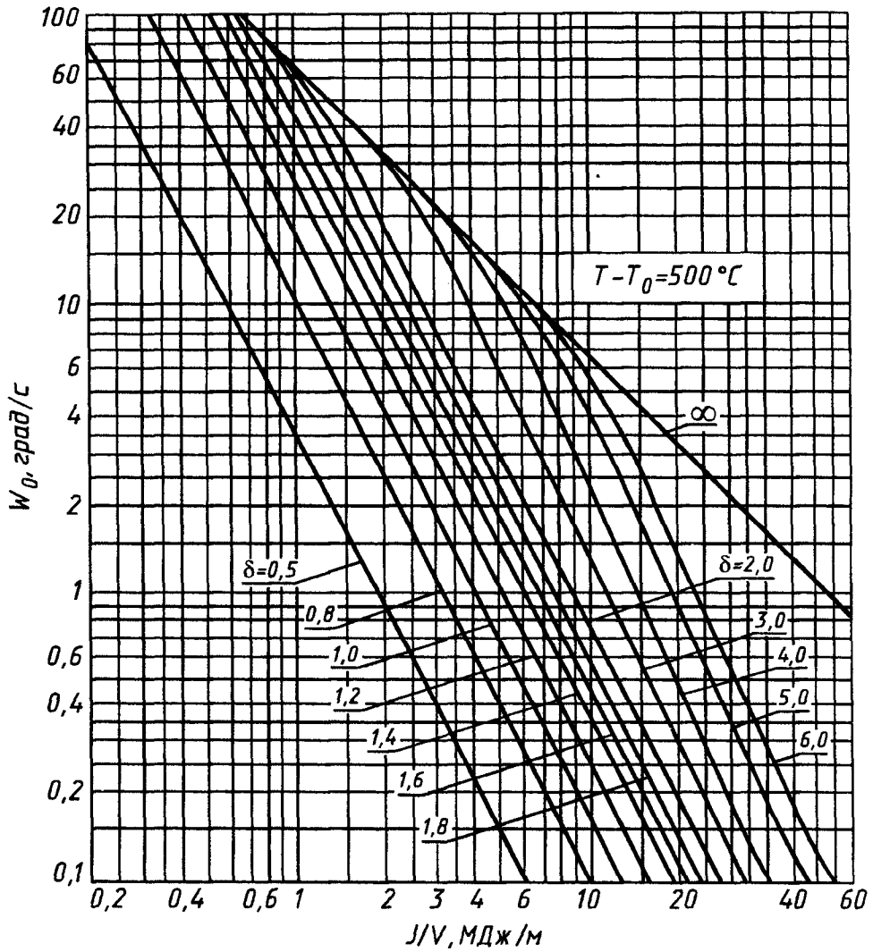
Номограмма для определения скорости охлаждения ЗТВ W_0 при наплавке валика на пластину
